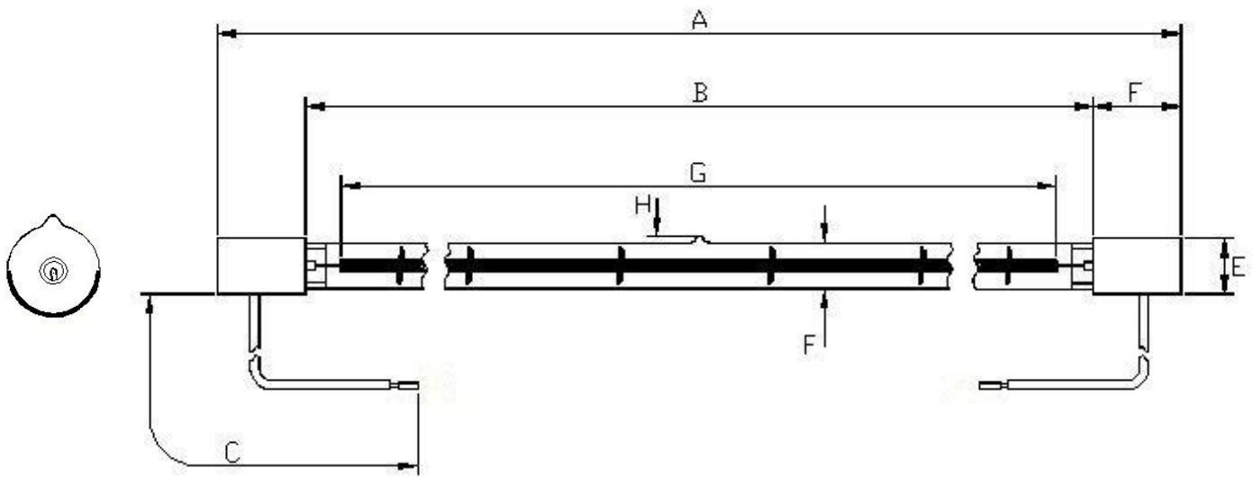
Dimensions
